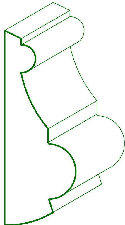
MC - 1469 1 1/4 X 3 1/2
