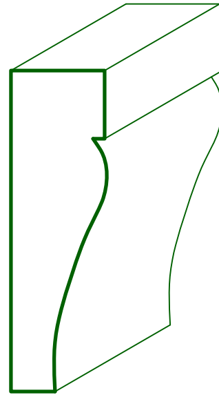
MC 4150 11/16 x 2 3/8
