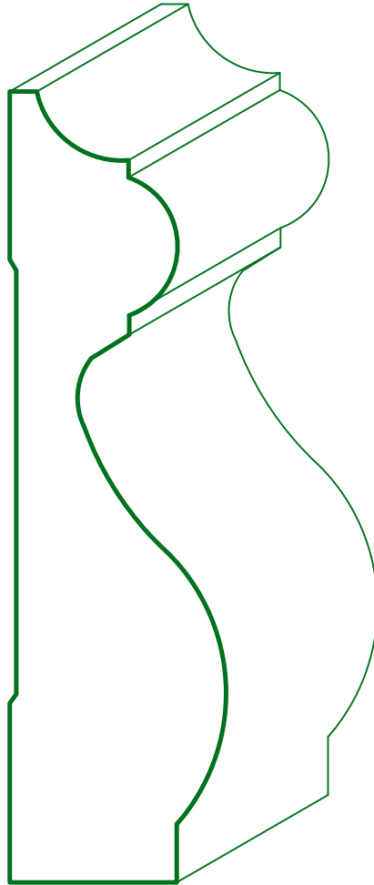
MC - 3706 1 1/4 X 4 1/2
