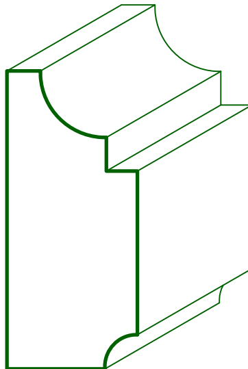
MC 4385 1 x 2 1/4
