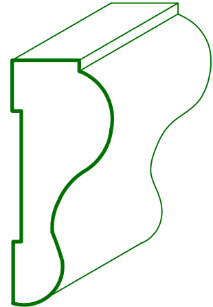
MC - 1077 13/16 X 1 7/8
