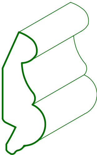
MC - 1340 3/4 X 2 1/16
