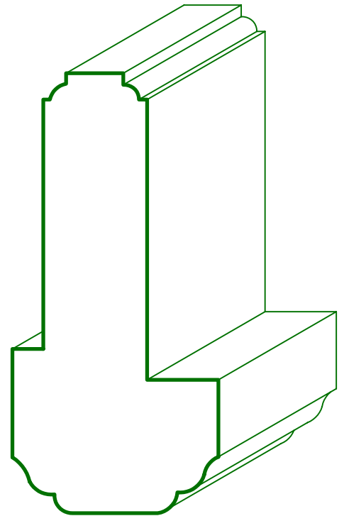
MC - 1974 3 1/4 X 1 1/2
