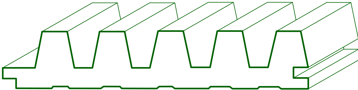
MC 4089 1 x 5 1/4
